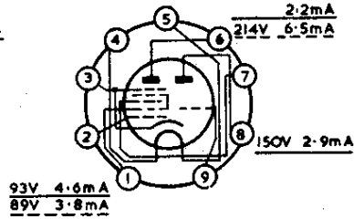
ECH81
