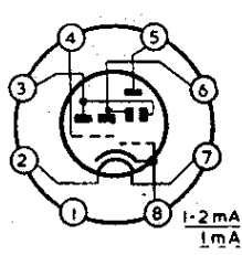
EM34
