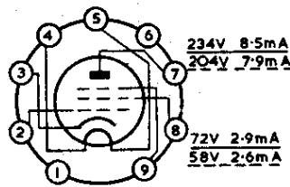
EF89
